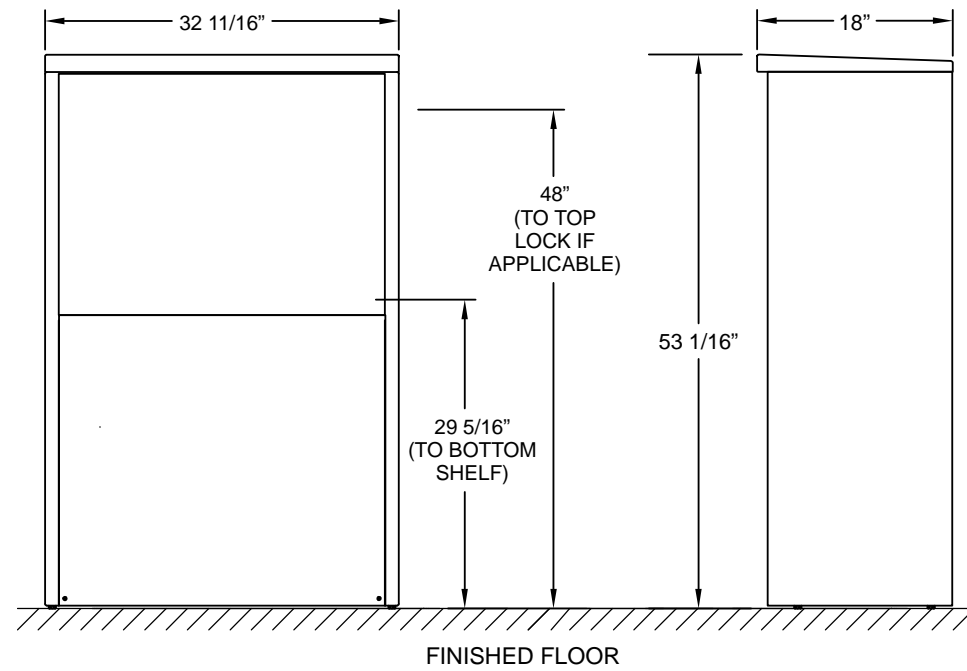
Elevation 1 - 4C06
